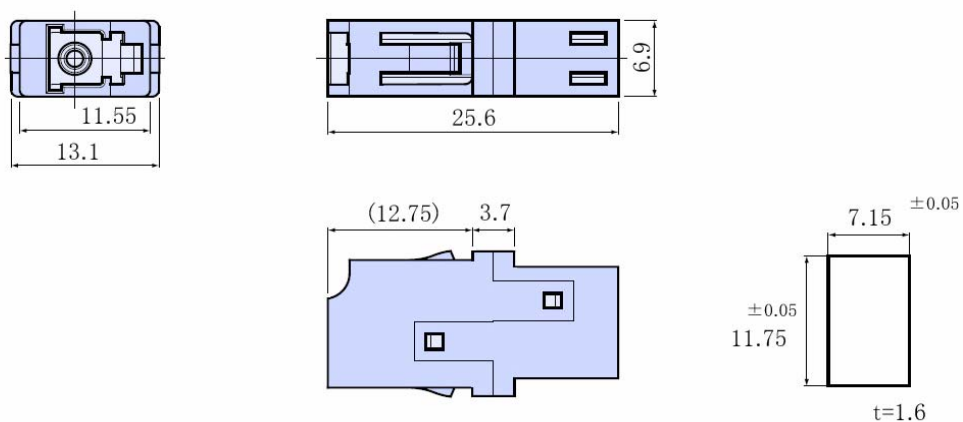
取付穴寸法
